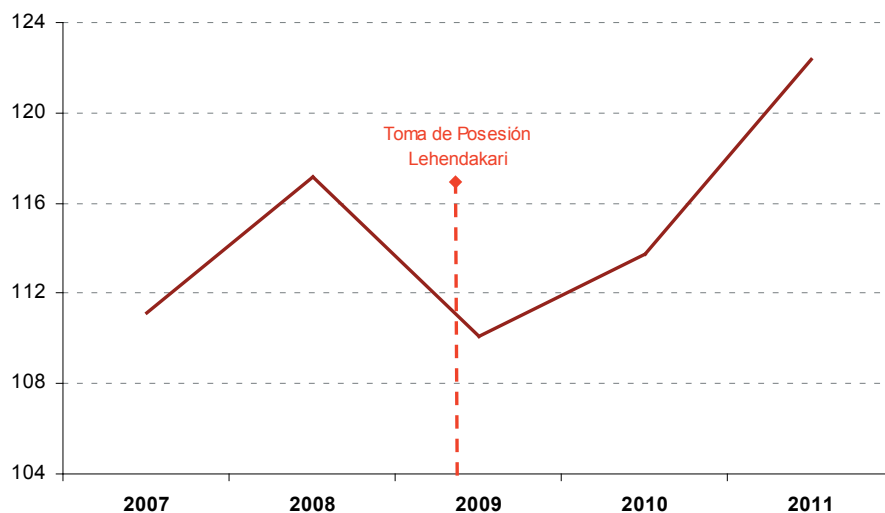
Evolución Índice de Producción Industrial - IPI (2007 - 2011)
