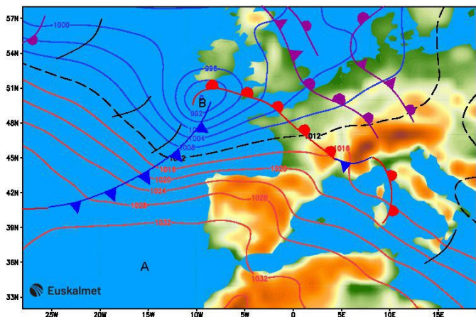
Fronteak eta Presioa itsas mailan (mb) 2026/01/08 12:00 Frentes y Presión nivel mar (mb)
