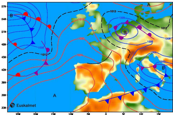
Fronteak eta Presioa itsas mailan (mb) 2026/01/10 12:00 Frentes y Presión nivel mar (mb)
